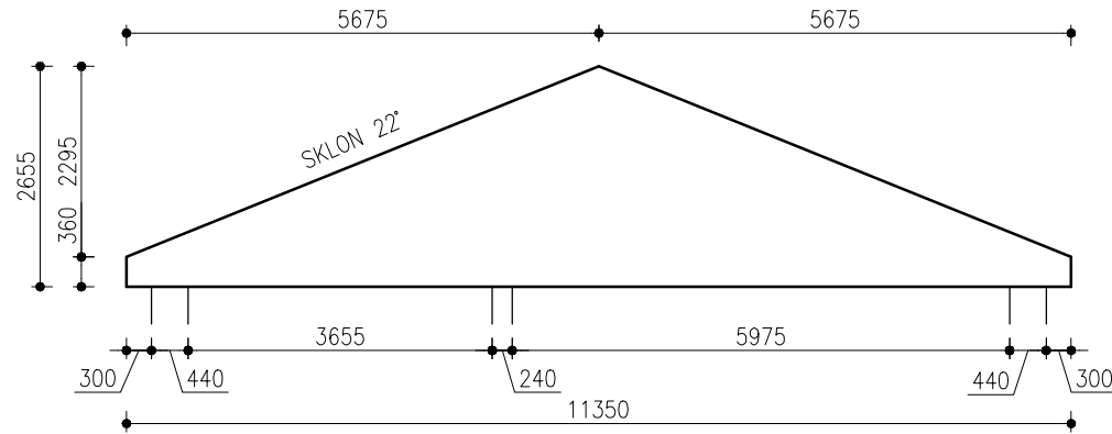
SCHEMA DŘEVĚNÉHO STYČNÍKOVÉHO VAZNÍKU
