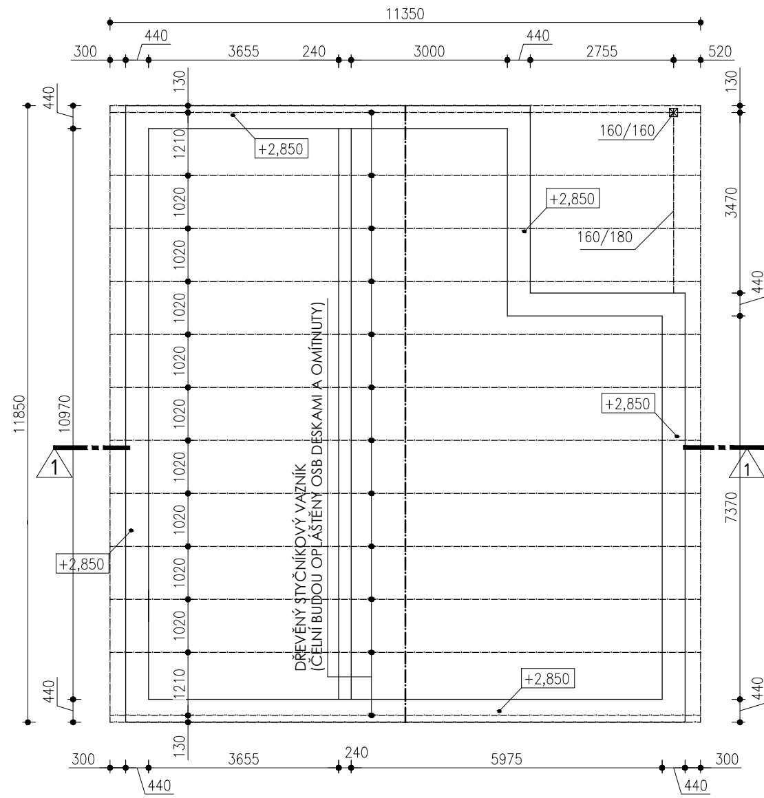
SCHEMA DŘEVĚNÉHO STYČNÍKOVÉHO VAZNÍKU
